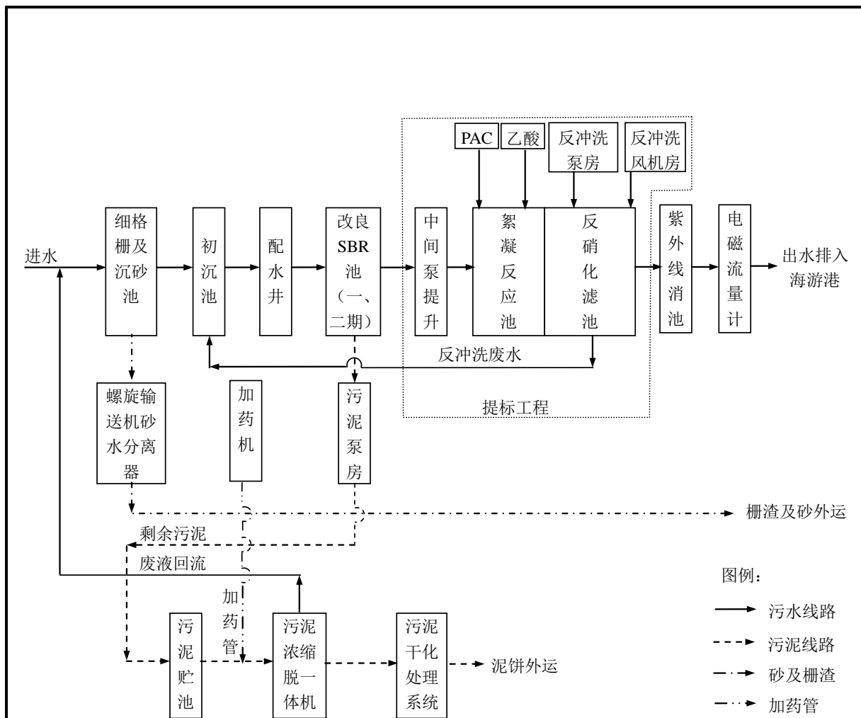
图 2-1 三门污水处理厂提标工程处理工艺流程图
