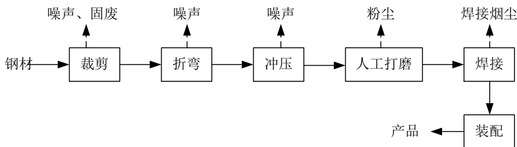
图 5-1 本项目工艺流程及产污节点图
